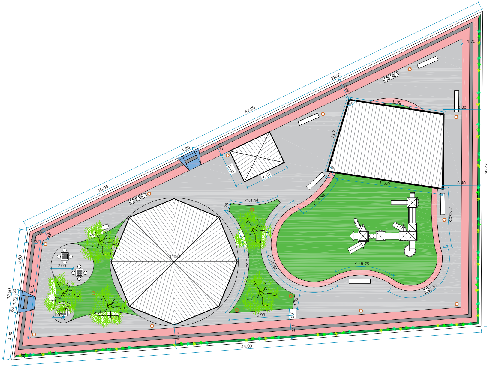
PLANTA DE COBERTA PRAÇA NOVA COREMAS ESCALA: 1/150
